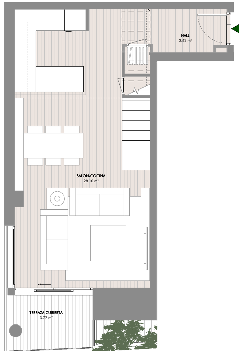
PLANTA 3ª PLANTA BAJA DUPLEX
