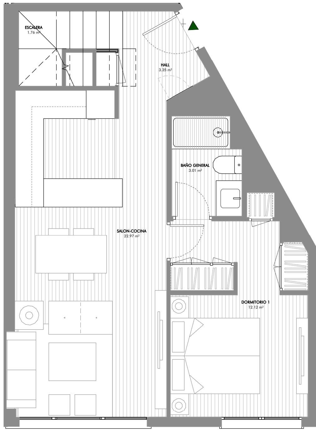
PLANTA 3º PLANTA BAJA DUPLEX
