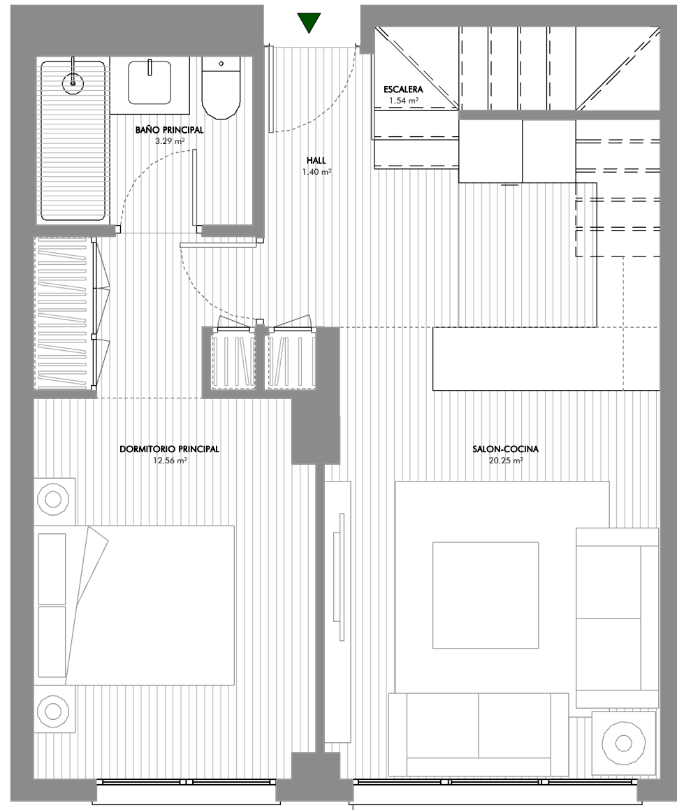
PLANTA 3º PLANTA BAJA DUPLEX
